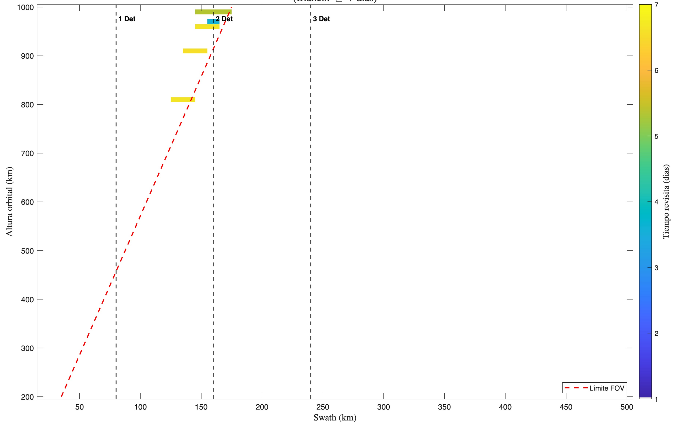
Tiempo Revisita - 3 Satellite(s); 1 Telescopio(s): Refractivo; Detector 3 (Blanco: \geq 7 días)
